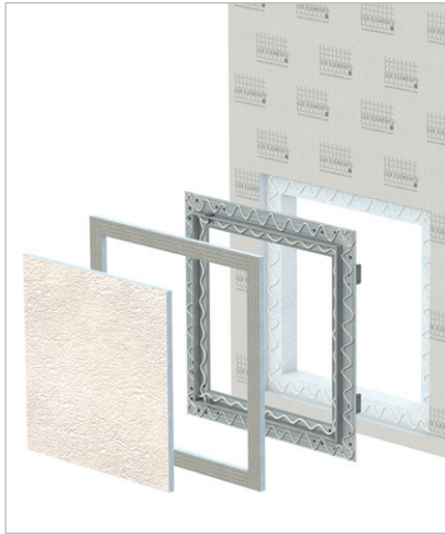
Application avec enduit : avec panneau frontal / pièces d'obturation sur cadre
