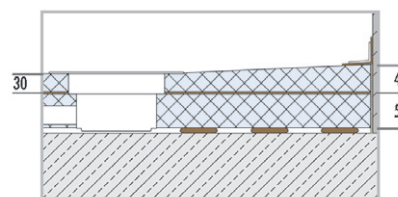
Siphon de sol horizontal avec élément support
