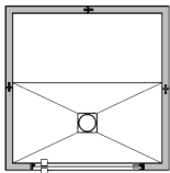
MODUL-CAB-Q – quadratische Kabine MODUL-CAB-Q 1180 MODUL-CAB-Q 1450
